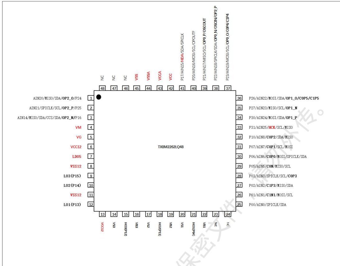
图 2 -TX8M2262LQ48 (LQFP48) 封装图
